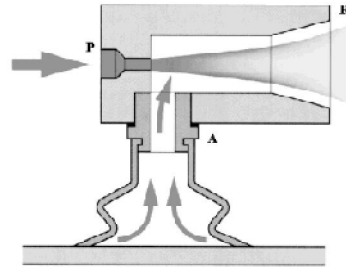
Ventouse de préhension
