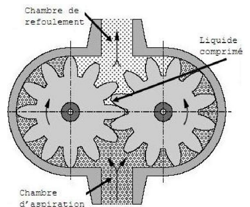
Moteur à engrenage
