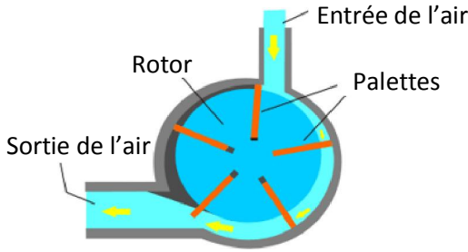
Moteur pneumatique à palettes
