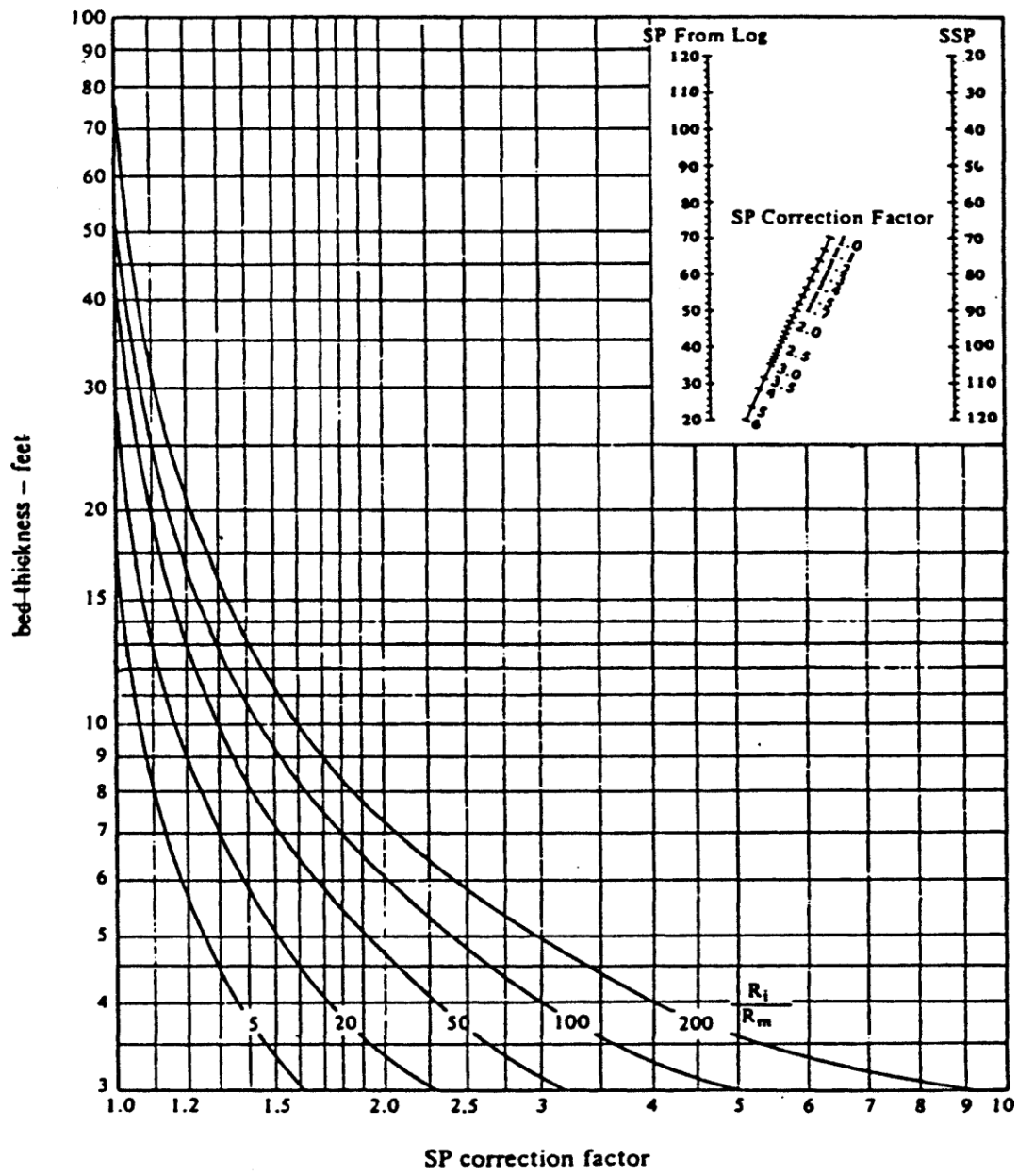
Abaque 6 : Correction de l'effet de banc pour le calcul de R_w , S_{pcor} = SP \times Cor. F.
