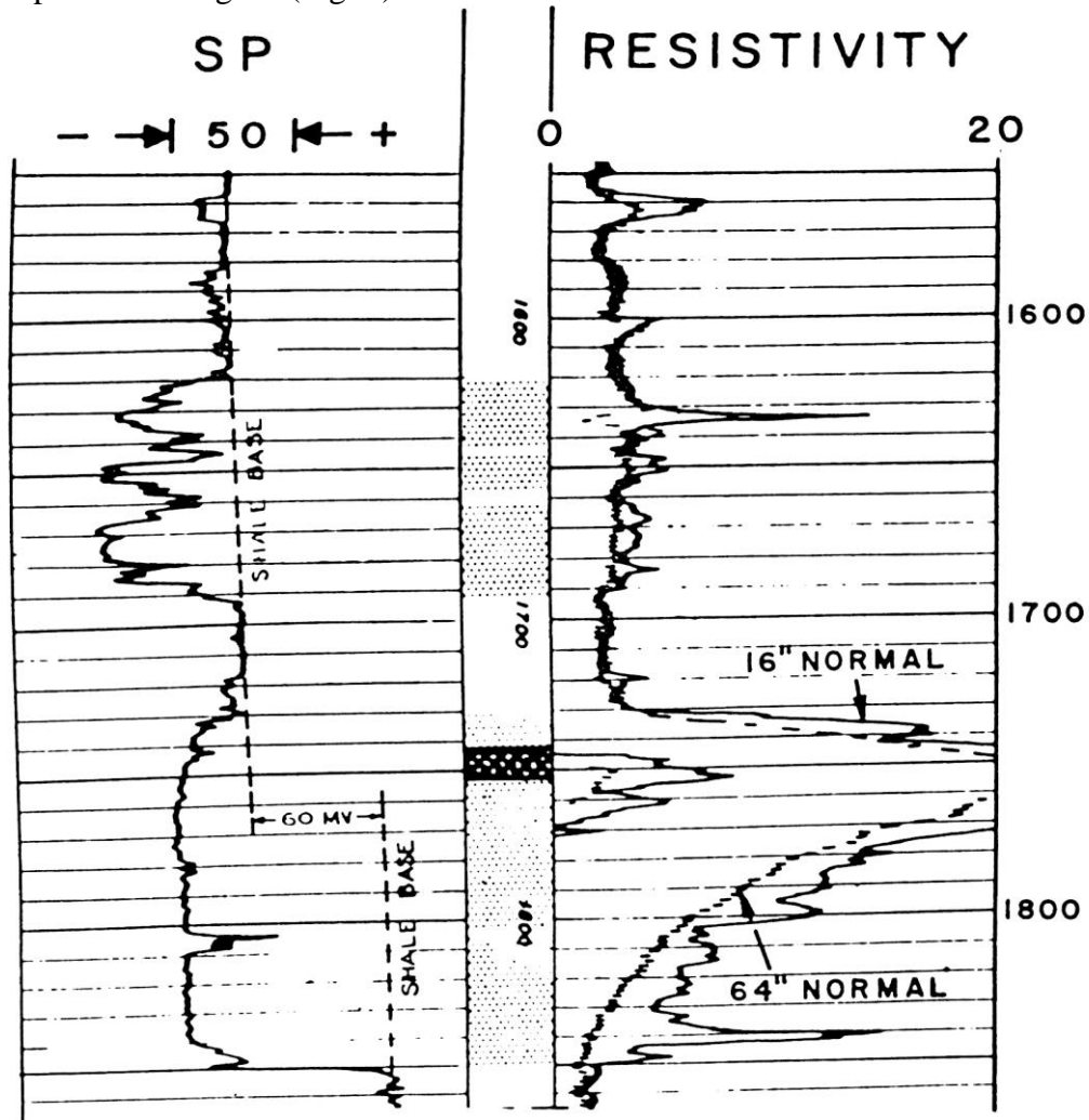
Fig 7. Changement de la ligne de base des argiles (D'après Guyod).
