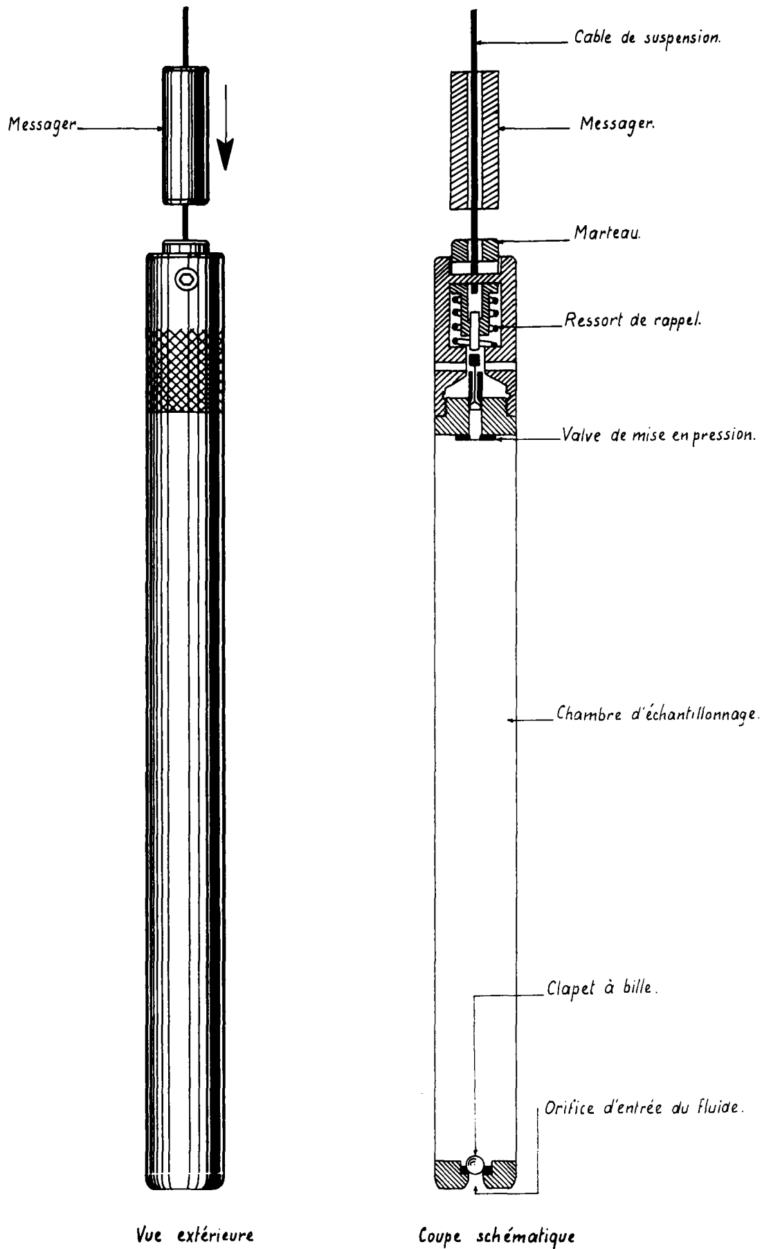
Fig. 2 : Exemple d'hydrocapteur descendu fermé, ouvert en profondeur. Hydrocapteur NEYRPIC (Documents NEYRPIC)
