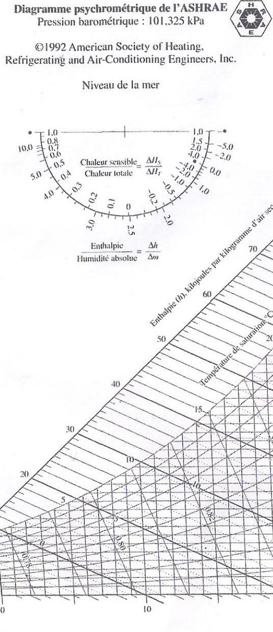
FIGURE A.30 Diagramme psychrométrique à 1 atm.
