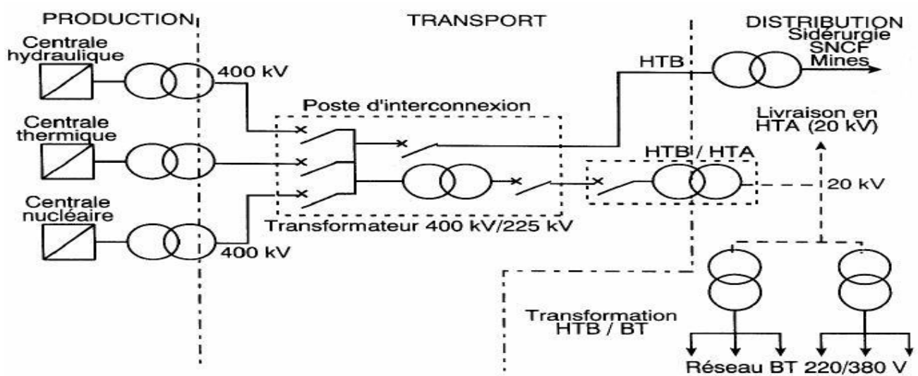
Schéma général de la production, du transport et de la distribution d'énergie électrique.
