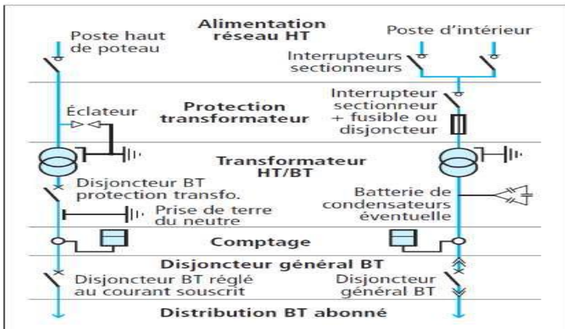
Fig. 1 : Structure générale d'un poste HTA/BT.
