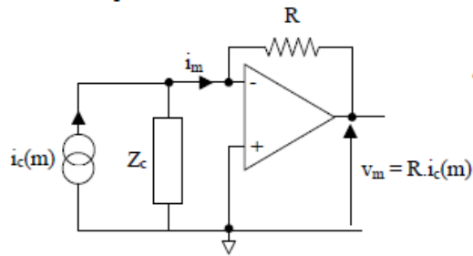
Figure 16. Convertisseur courant/tension
