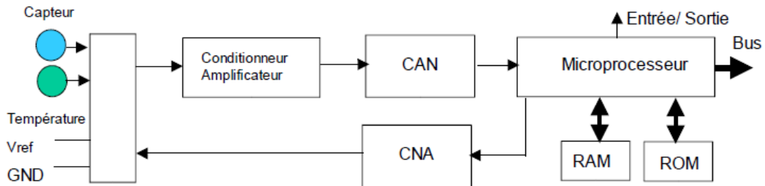
Figure 11. Structure complexe d'un capteur intelligent
