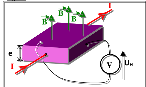
Fig. 5 : L'effet Hall
