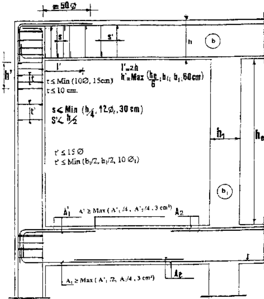
Détail d'un cours d'armatures transversales de la zone nodal.
