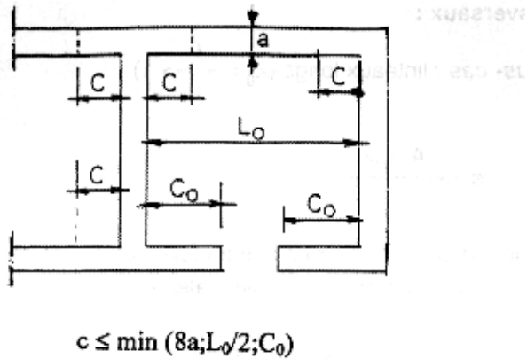
Fig. 7.9 : Prise en compte des murs en retour
